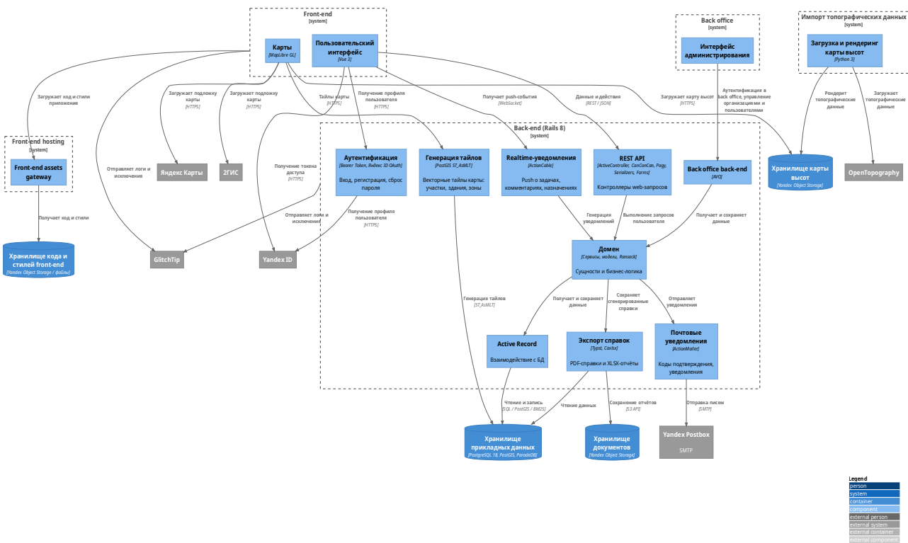
Рис. 1: Архитектурная схема компонентов и слоёв ПО
